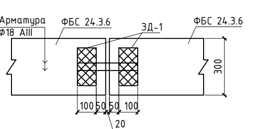
ПЛАН объединения блоков ФБС
